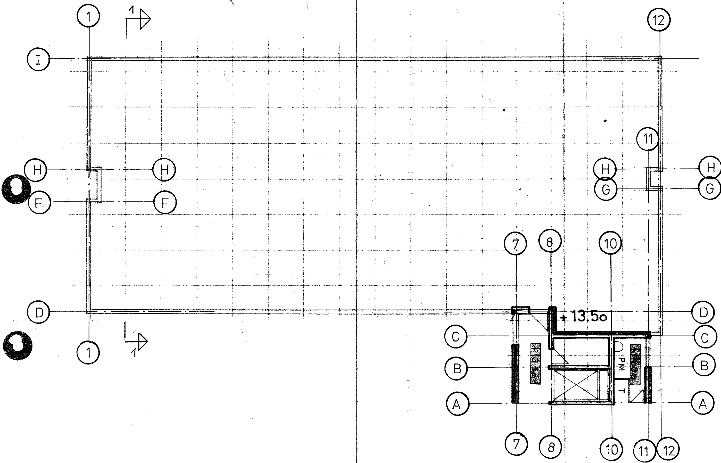
MÜ - EN DACHGRUNDRISS 1:100
